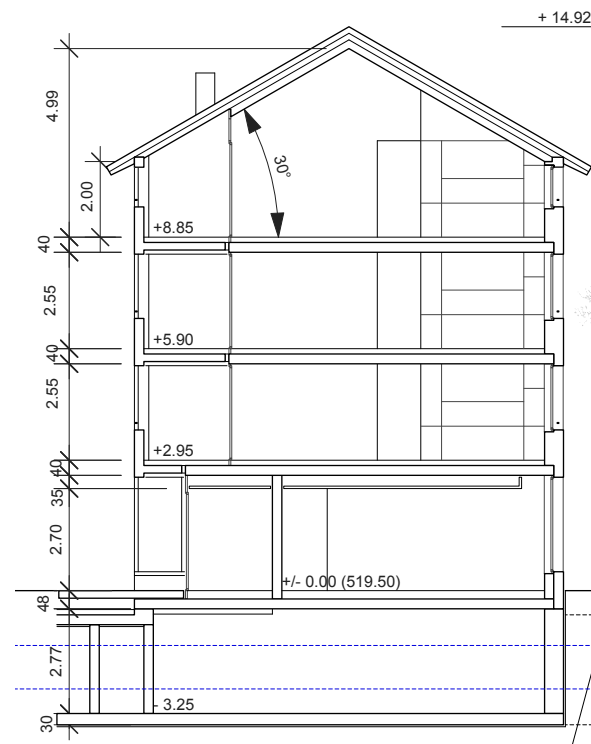
Haus 4 Querschnitt
