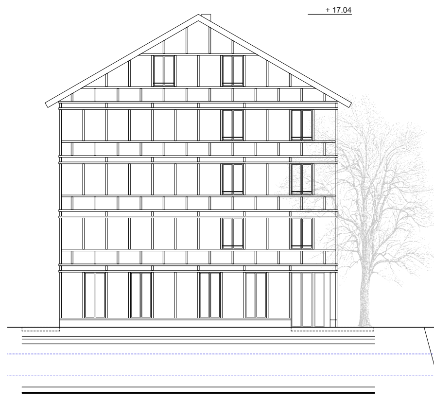
Haus 3 Nordost
