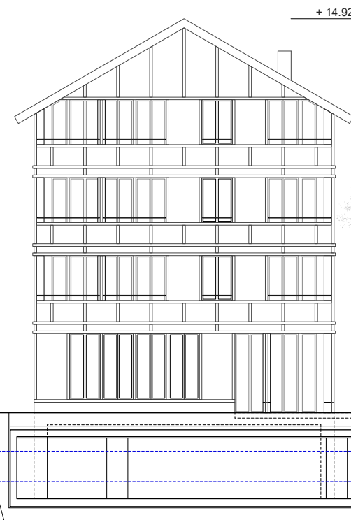
Haus 4 Südwest
