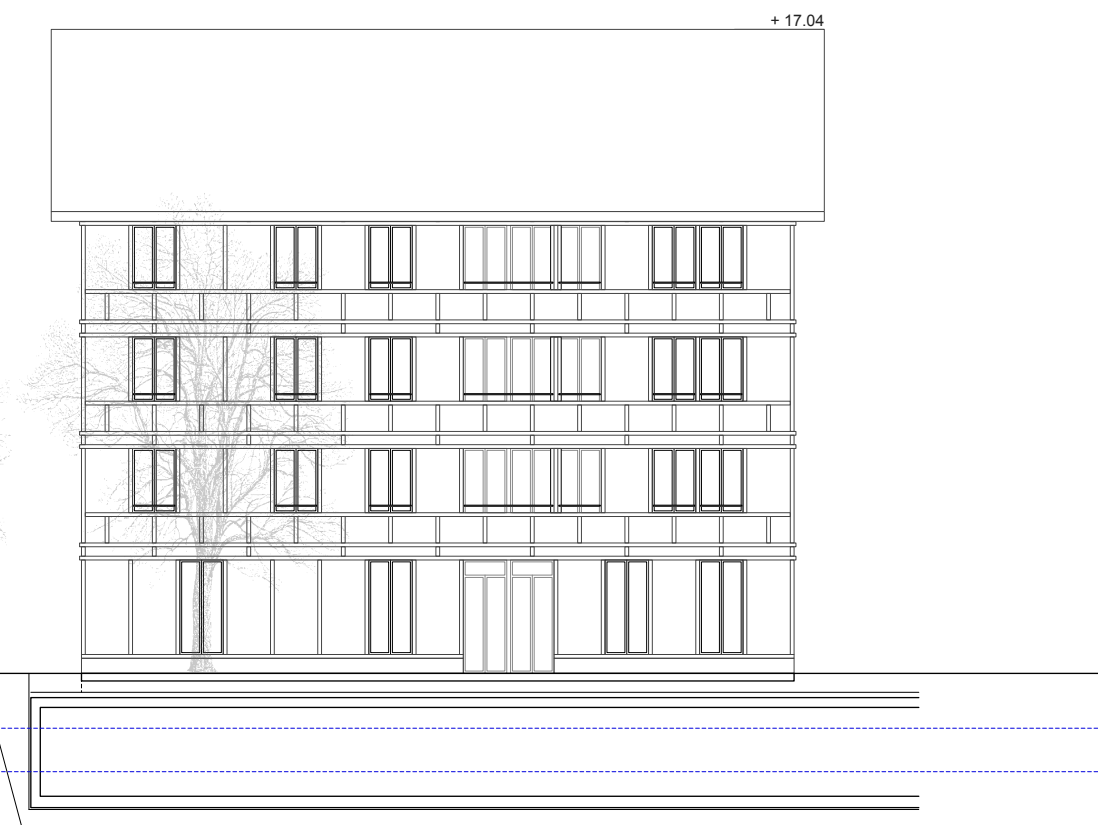
Haus 3 Südost
