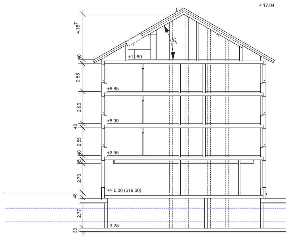
Haus 3 Querschnitt
