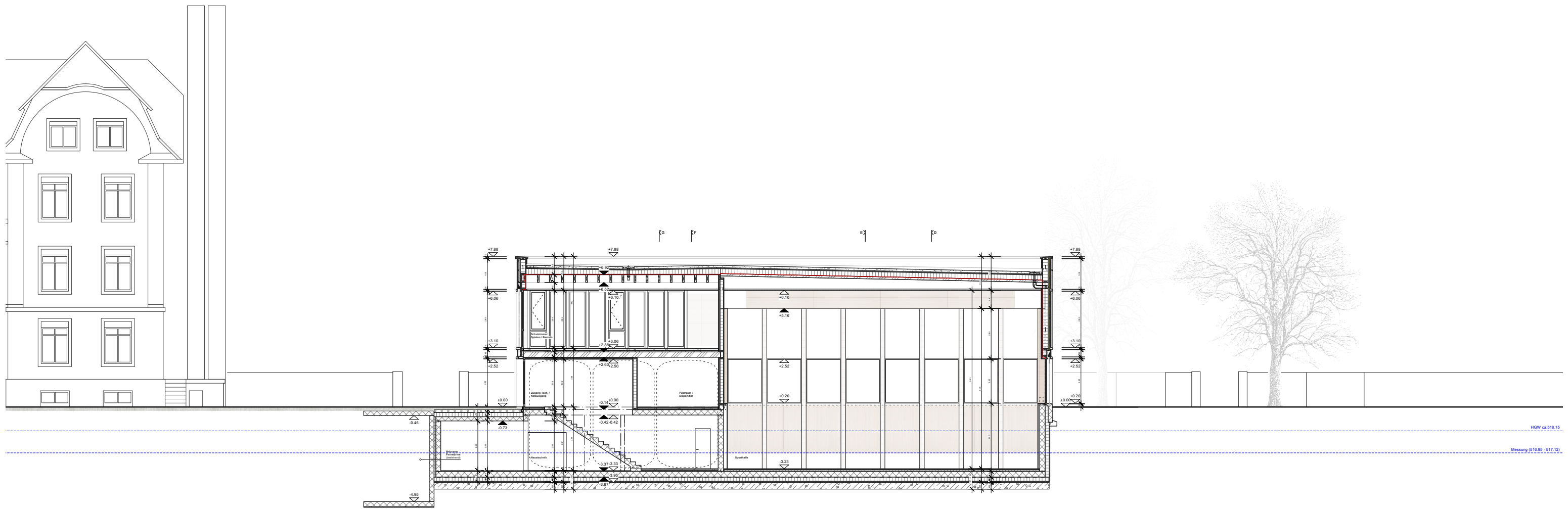
Schnitt C-C
